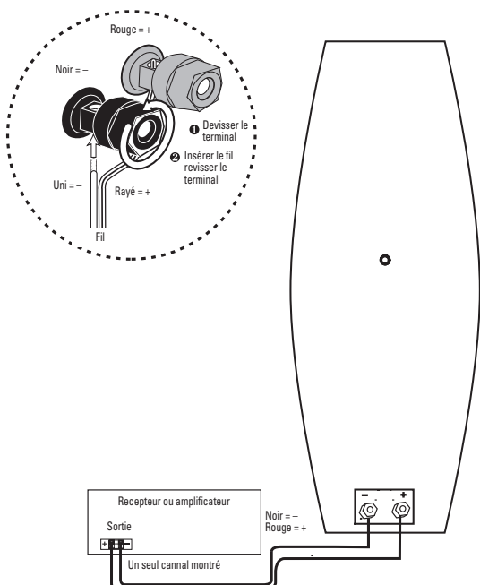
Figure 4. Le schéma de câblage indique les connexions de polarité pour un canal d'un système de cinéma à domicile.
