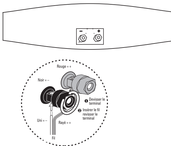
Figure 5. Les borniers des enceintes satellites et de l'enceinte centrale peuvent être connectés de plusieurs façons, par exemple avec cosses ou fils nus (comme sur l'illustration).
